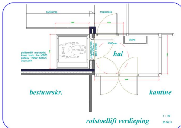
Situatie plaatsing lift
